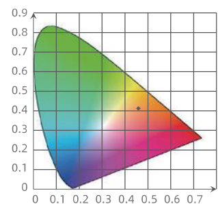
CIE 1931 x y Chromaticity Diagram
